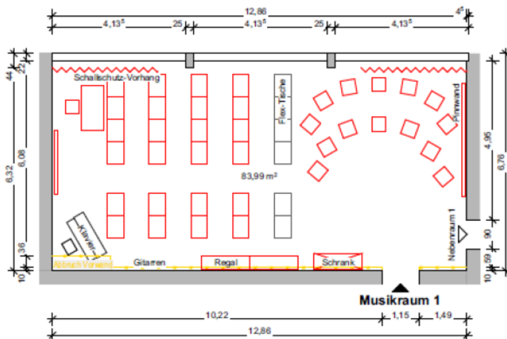
Grundrissbeispiel (Wentorf)
